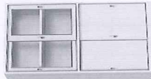
MY-OC-15 H1850*W900*D400mm
